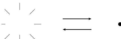
図 7.2: makeVertex ・ removeVertex
